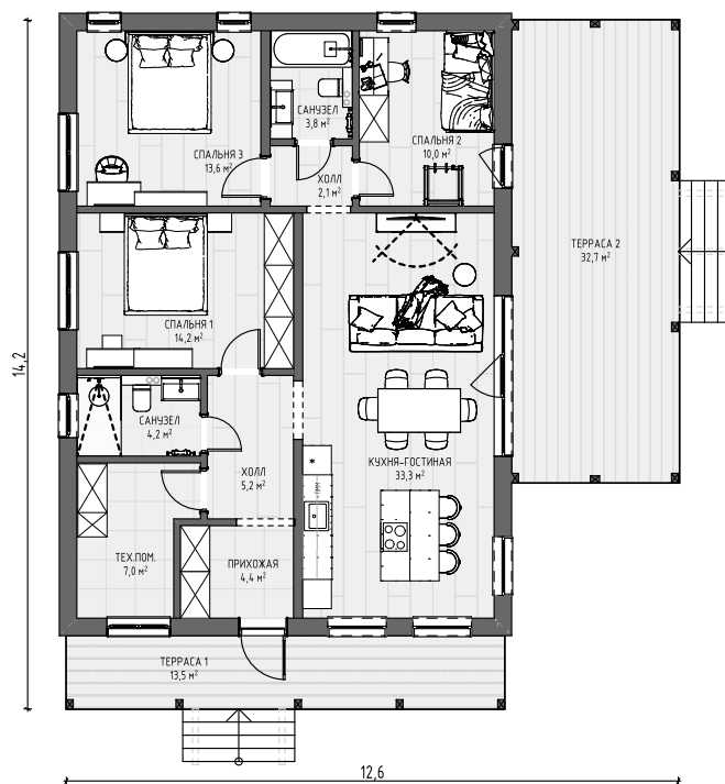
Планировка № 2
