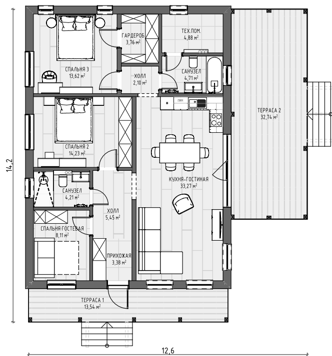
Планировка № 1
